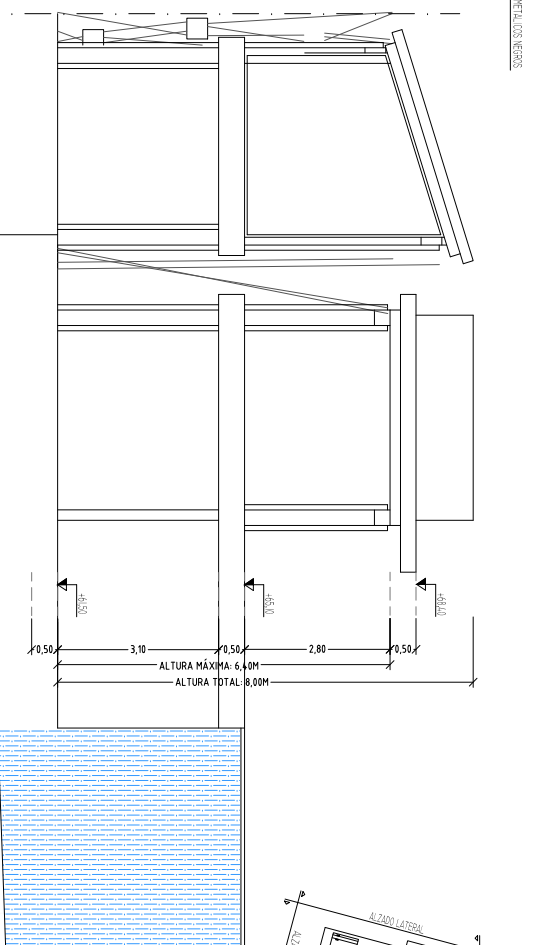
ALZADO COMEDOR-COCINA
